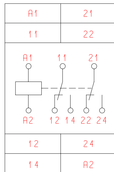
Bild 2: Anschluss RH 32
