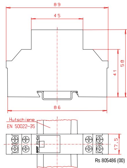
Bild 4: Maßbild
