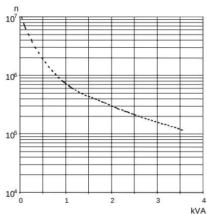
Bild 2: Kontaktelebensdauer in Abhängigkeit von der Schaltleistung bei ohmscher Wechselspannungsbelastung
