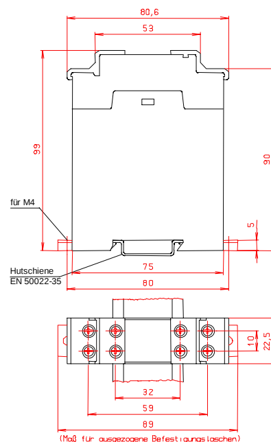
Bild 1: Maßbild RH 32
