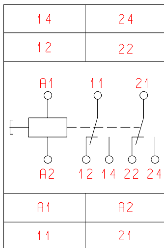
Bild 3: Anschluss
